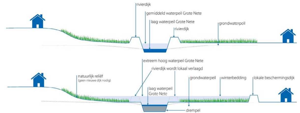
Afb. 8.1. Het herstel van de winterbedding in het kader van het Sigmaplan. Boven toont de bedding voor herstel. Onder na herstel.
